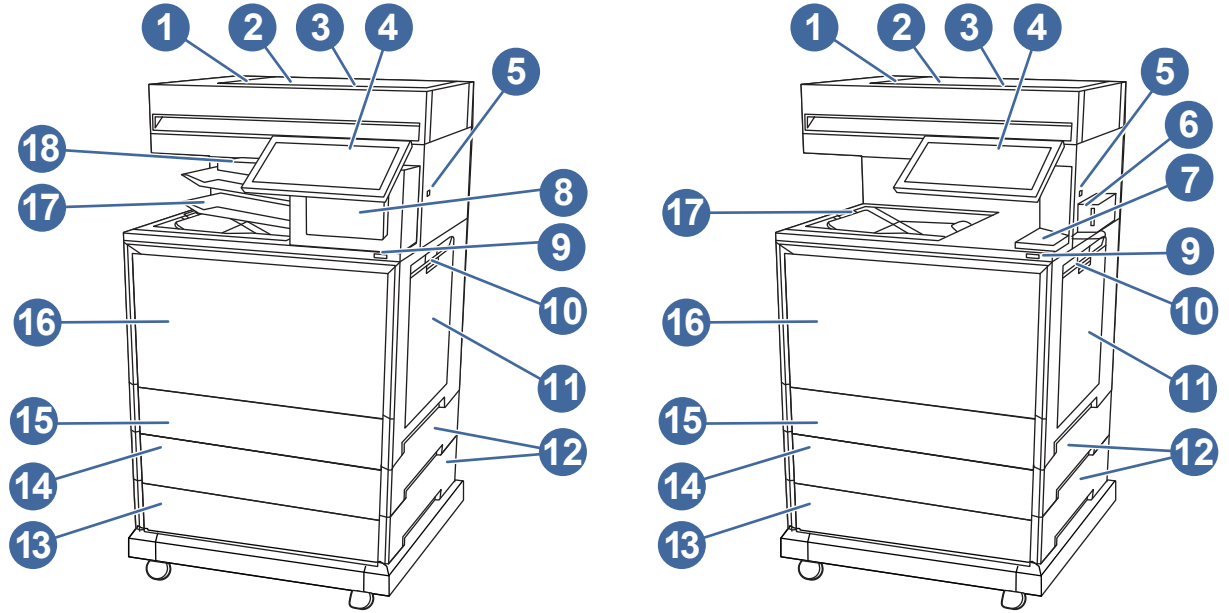
그림 17 프린터 전면 보기 -z 및 zs 모델(옵션 용지함 포함)
