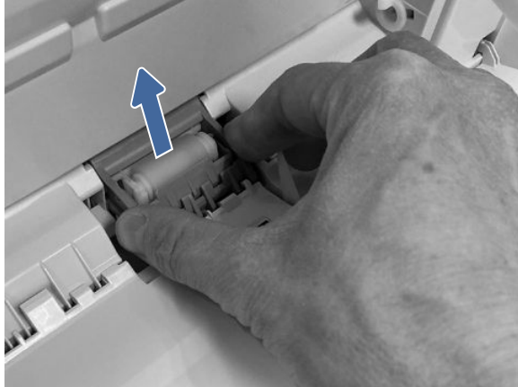
그림 9-7 분리 롤러 어셈블리 들어 올리기
