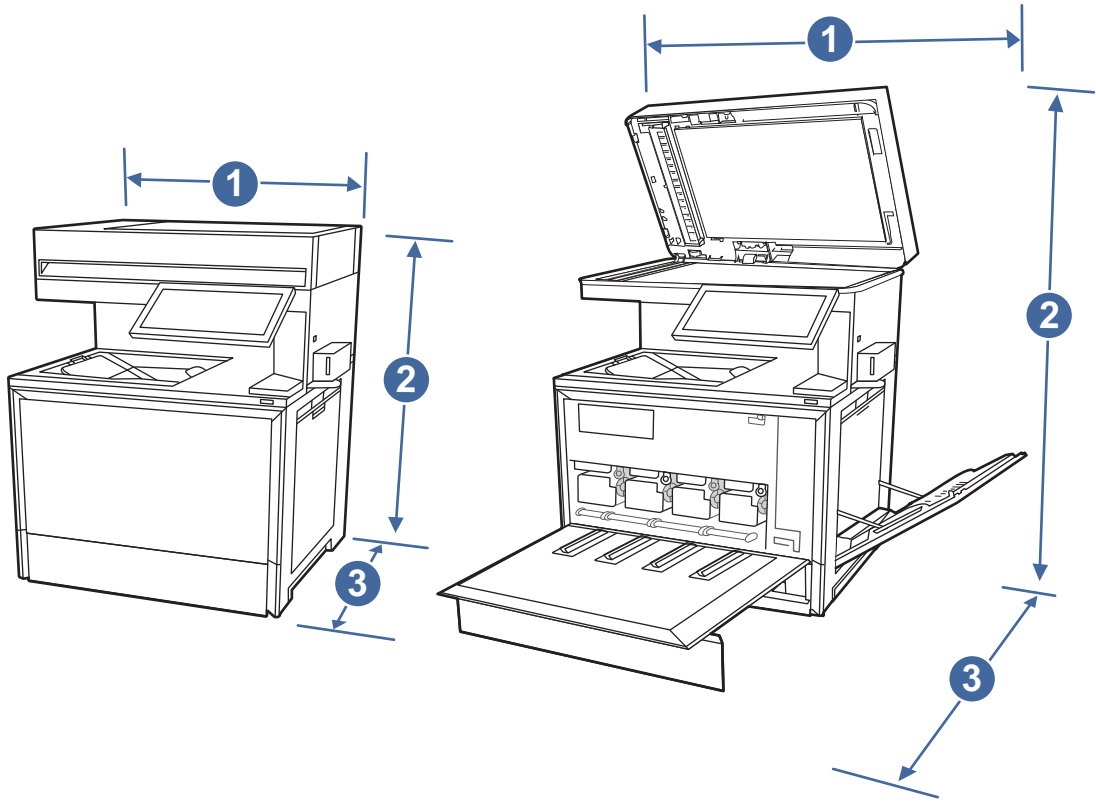
그림 1-11 프린터 크기(z 모델)
