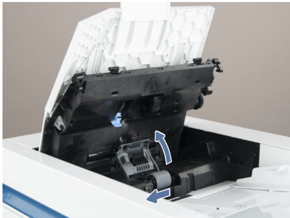
그림 9-4 분리 롤러 덮개 풀기
