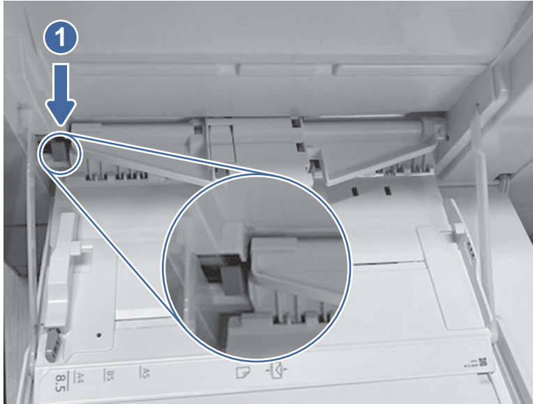
그림 9-5 픽업 롤러 어셈블리 탭 찾기
