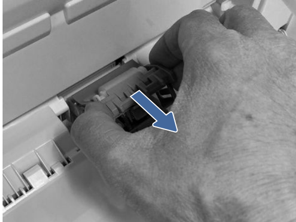
그림 9-8 분리 롤러 어셈블리 분리
