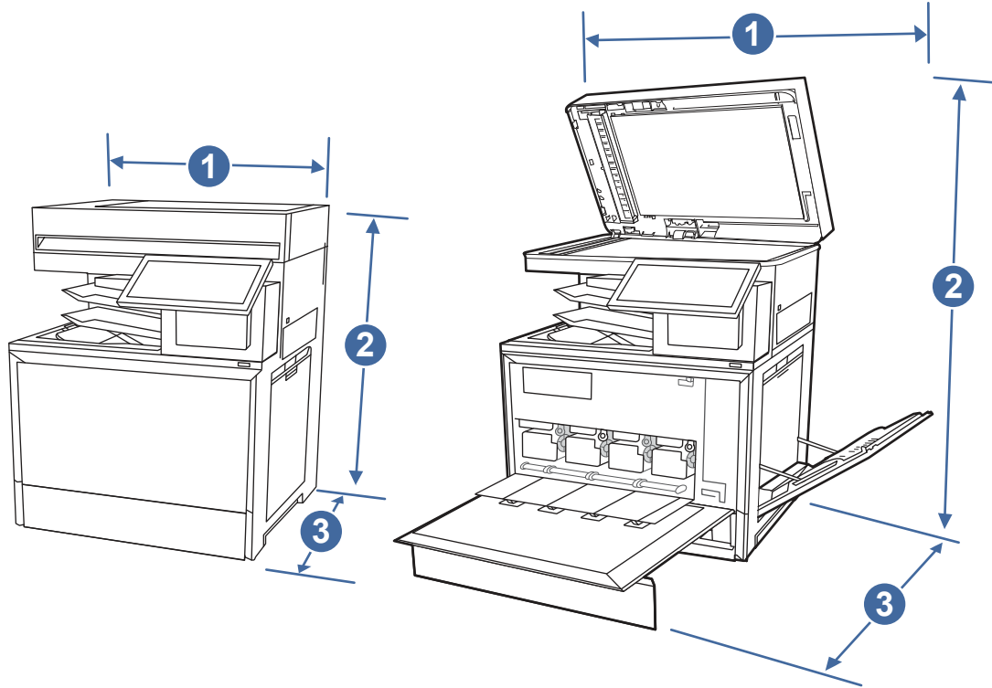
그림 1-12 프린터 크기(zs 모델)
