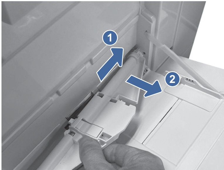
그림 9-6 픽업 롤러 어셈블리 분리
