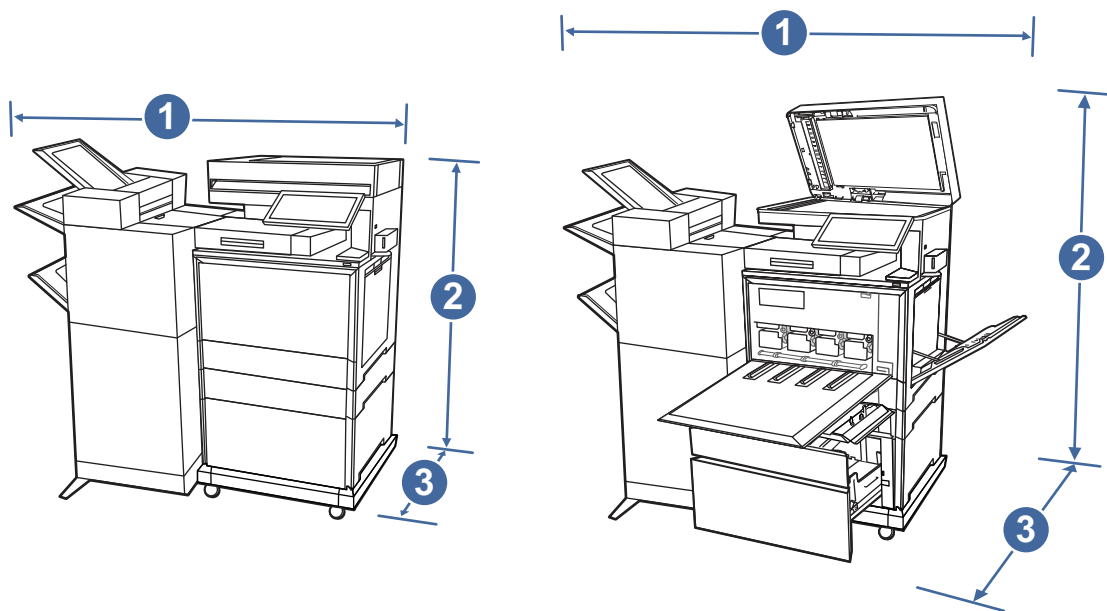
图 1-12 打印机尺寸 ( zfw+ 型号 )
