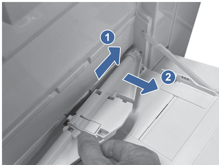
图 9-16 卸下拾纸轮组合件
