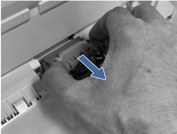
图 9-18 卸下分纸轮组合件
