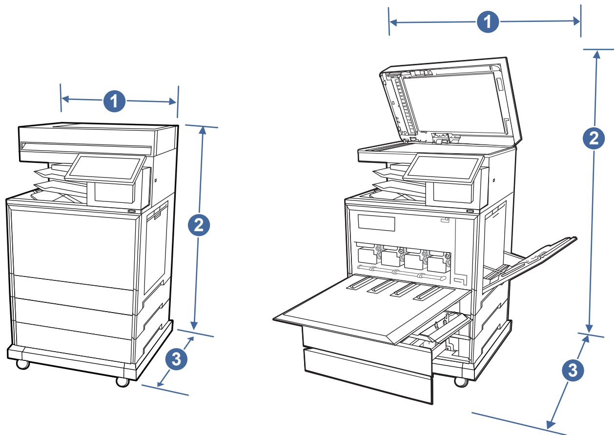
图 1-11 打印机尺寸 ( zfsw 型号 )
