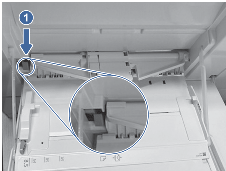
图 9-15 找到拾纸轮组合件压片
