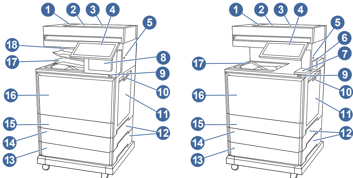
图 1-6 打印机前视图 - dn、zf 和 zfsw 型号
