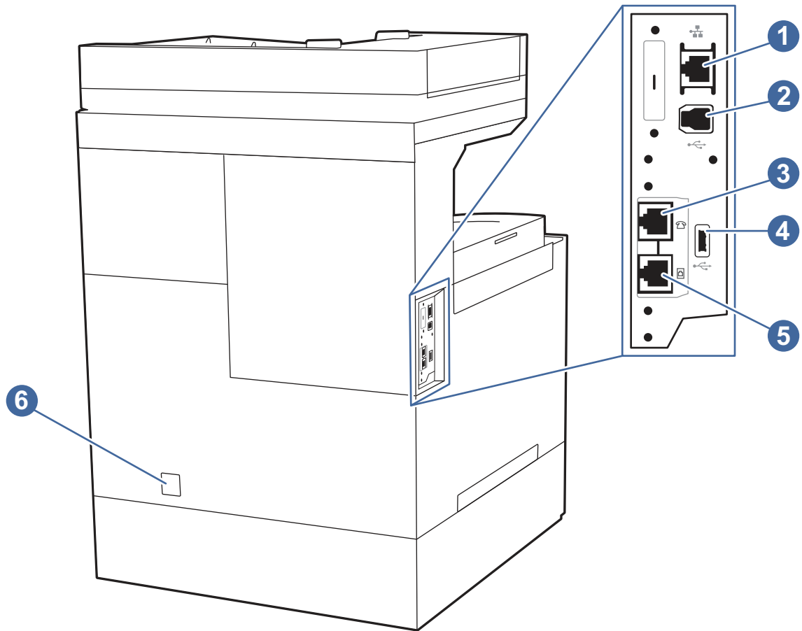
图 1-8 打印机后视图
