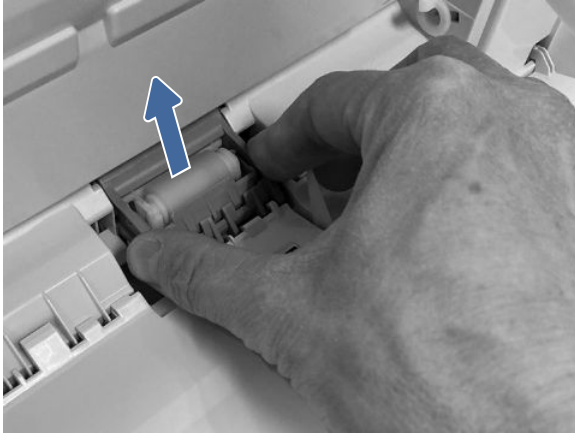
图 9-17 抬起分纸轮组合件
