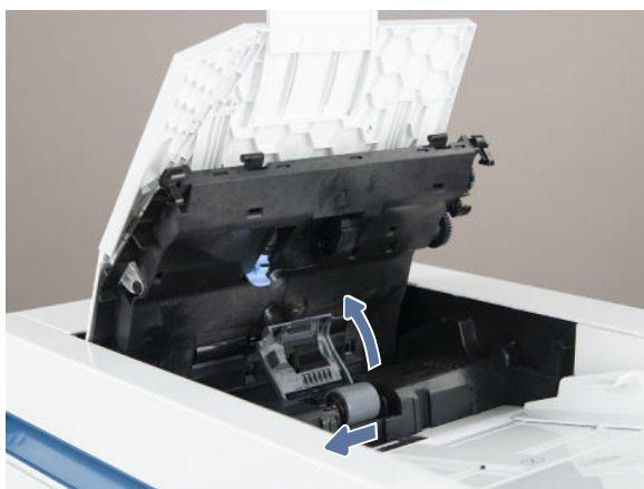
图 9-14 卸下分纸轮盖板
