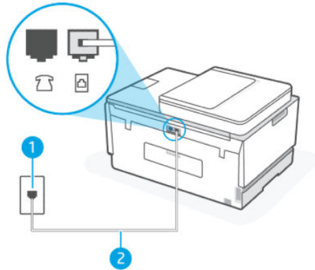
Abbildung 6-1 Rückansicht des Druckers
