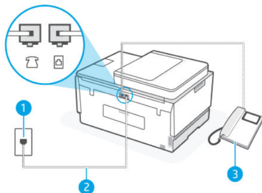
Abbildung 6-4 Rückansicht des Druckers
