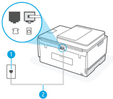
Abbildung 6-5 Rückansicht des Druckers
