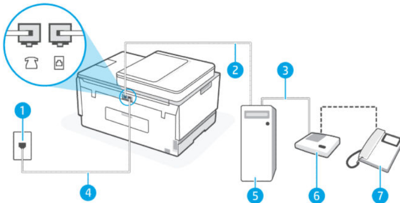
Abbildung 6-13 Rückansicht des Druckers
