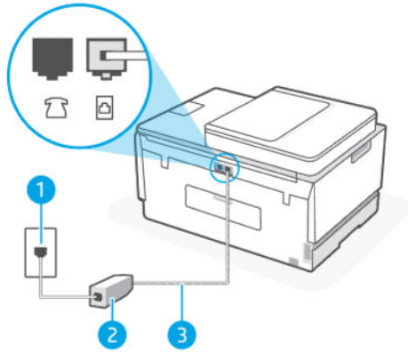
Abbildung 6-2 Rückansicht des Druckers
