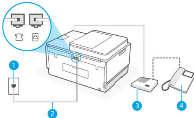
Abbildung 6-11 Rückansicht des Druckers
