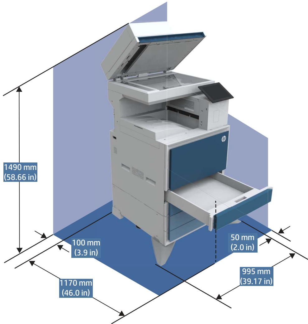
그림 110 프린터 및 이종 카세트 공급기 크기(완전히 열린 경우)
