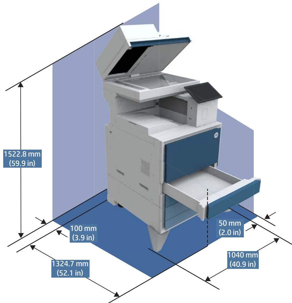
図 1-10 プリンタとデュアルカセットフィーダーの寸法 (完全に開いた状態)
