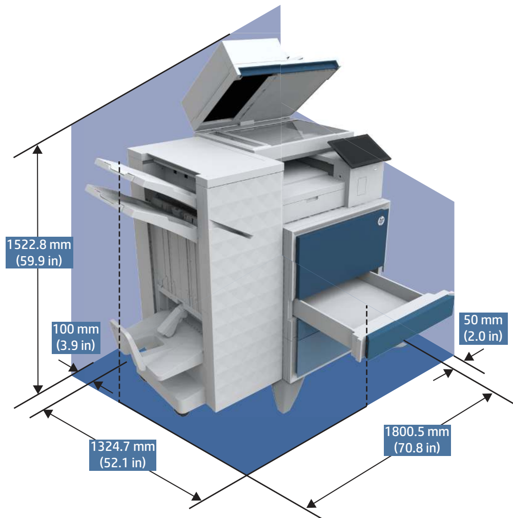
図 1-12 プリンタ、ブックレットフィニッシャ、および2K大容量給紙寸法 (完全に開いています)
