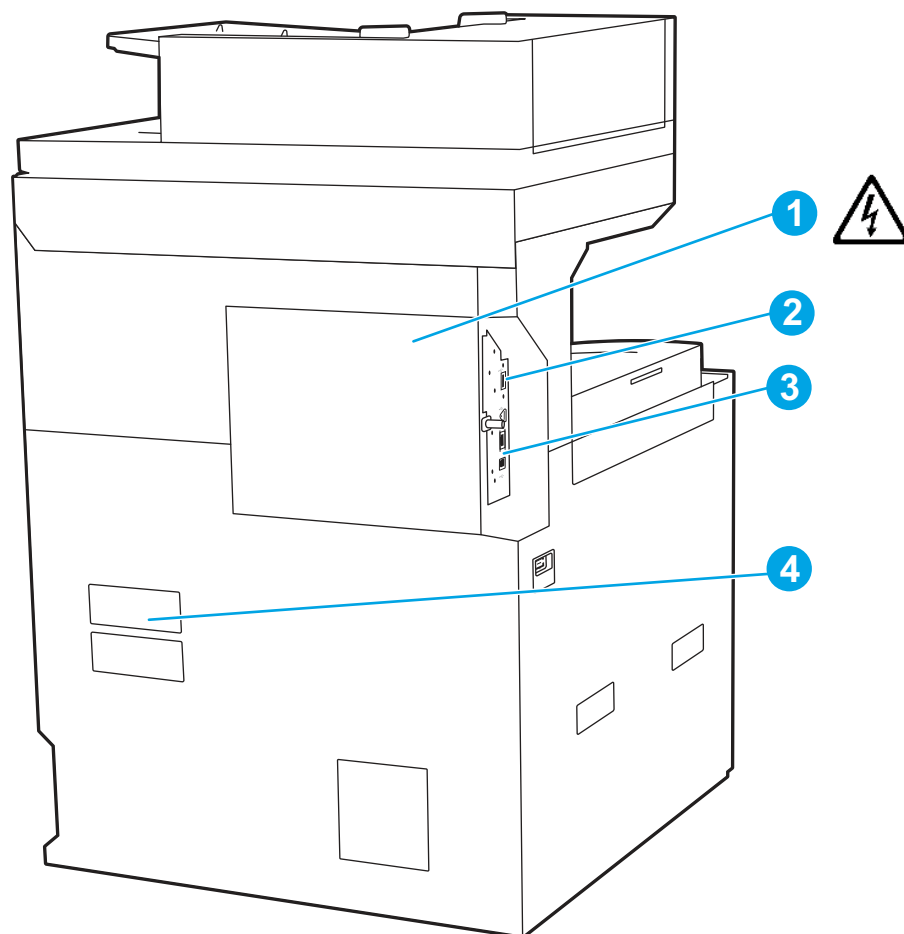
図17 プリンタの背面図
