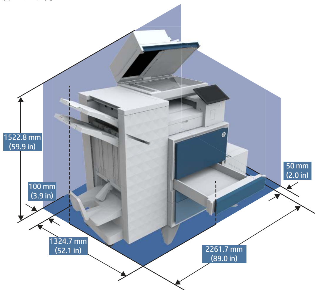
図 1-13 プリンタ、ブックレットフィニッシャ、2K大容量給紙、および側面の大容量給紙寸法 (完全に開いています)
