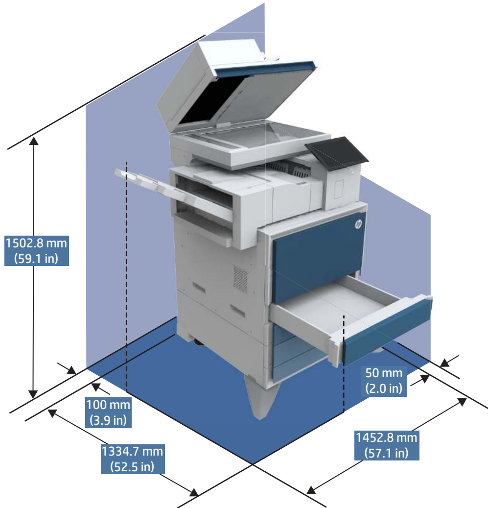
図 1-11 プリンタ、デュアルカセットフィーダー、および内部フィニッシャの寸法 (完全に開いた状態)
