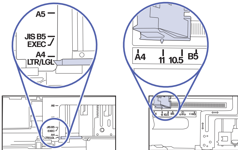
図 9-9 カセットトレイのサイズマーク
