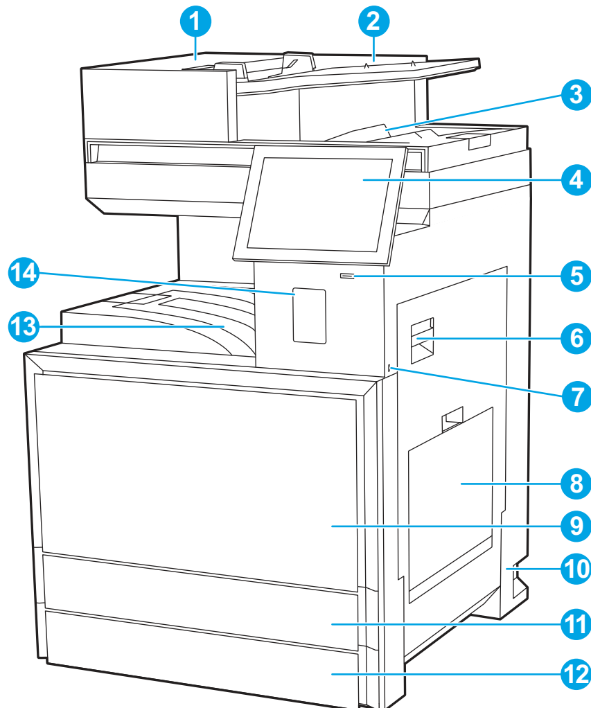
図 1-6 プリンタ前面図
