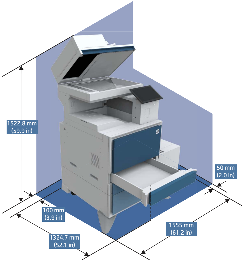
図 1-14 プリンタ、2K 大容量給紙、および側面の大容量給紙寸法 (完全に開いています)
