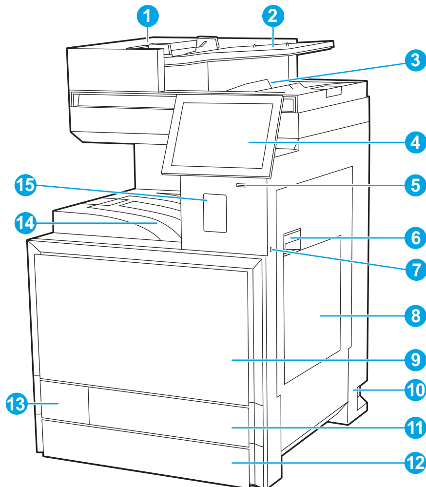
图 1-6 打印机前视图
