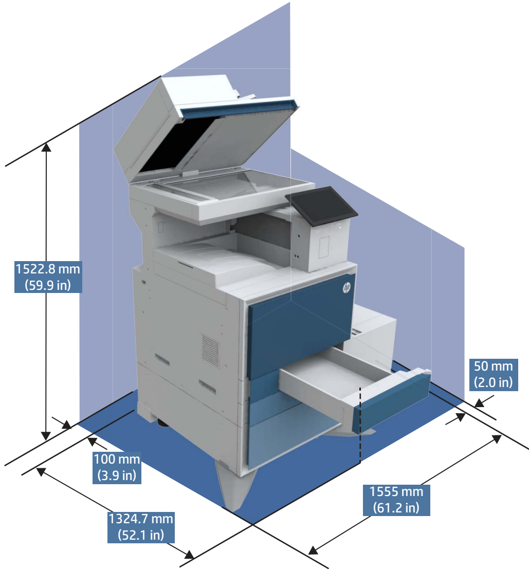
图 1-14 打印机、2K 大容量输入和侧面大容量输入尺寸 (完全打开)
