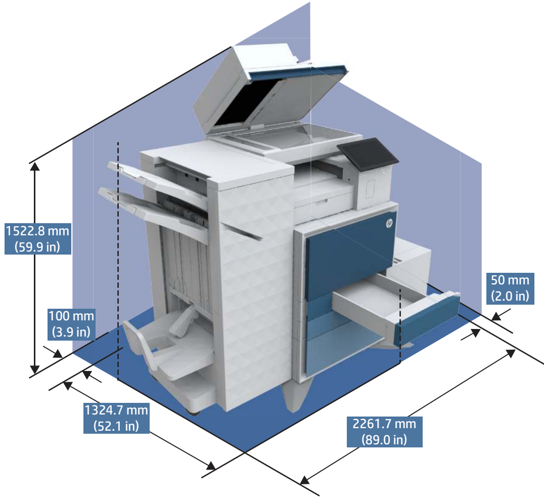
图 1-13 打印机、小册子装订器、2K 大容量输入和侧面大容量输入尺寸 (完全打开)
