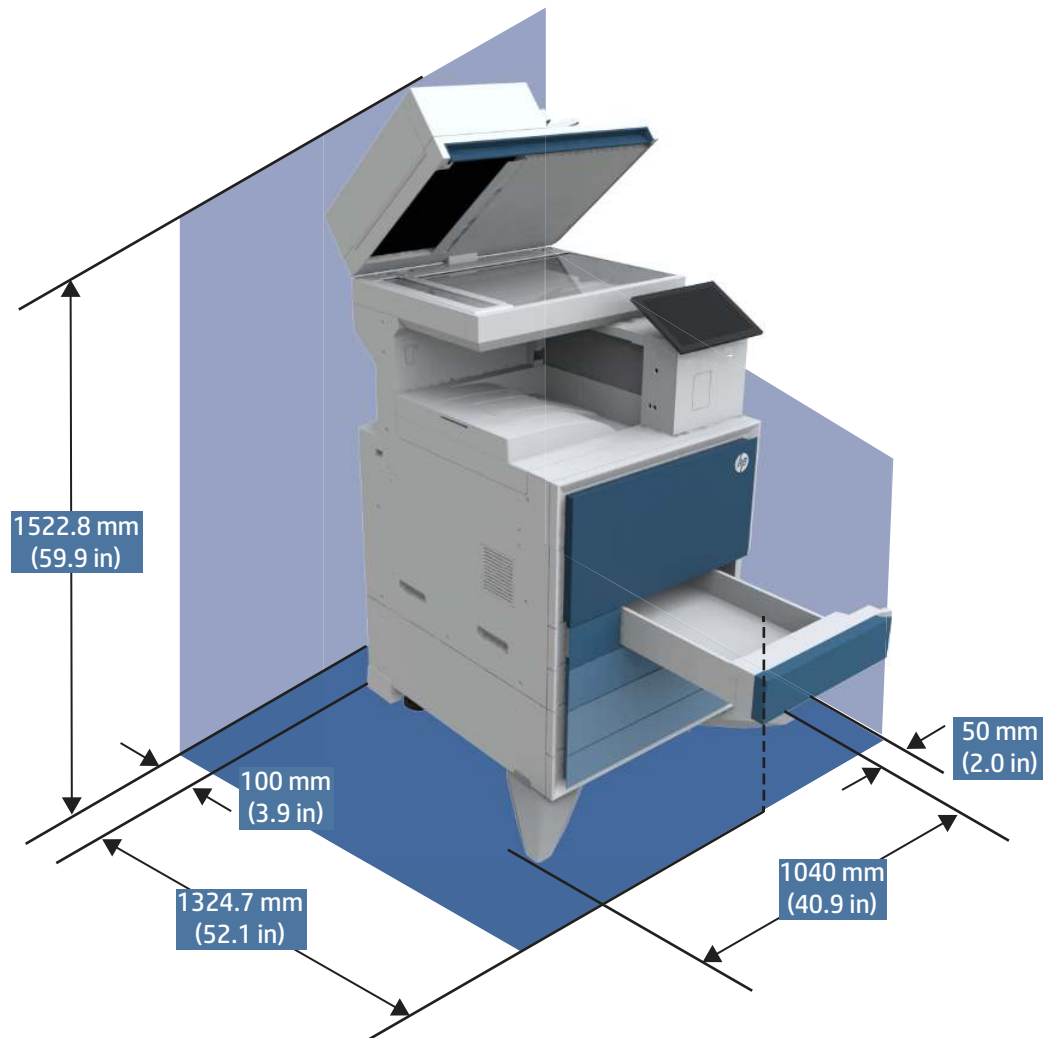
그림 1-10 프린터 및 이종 카세트 공급기 크기(완전히 열린 경우)
