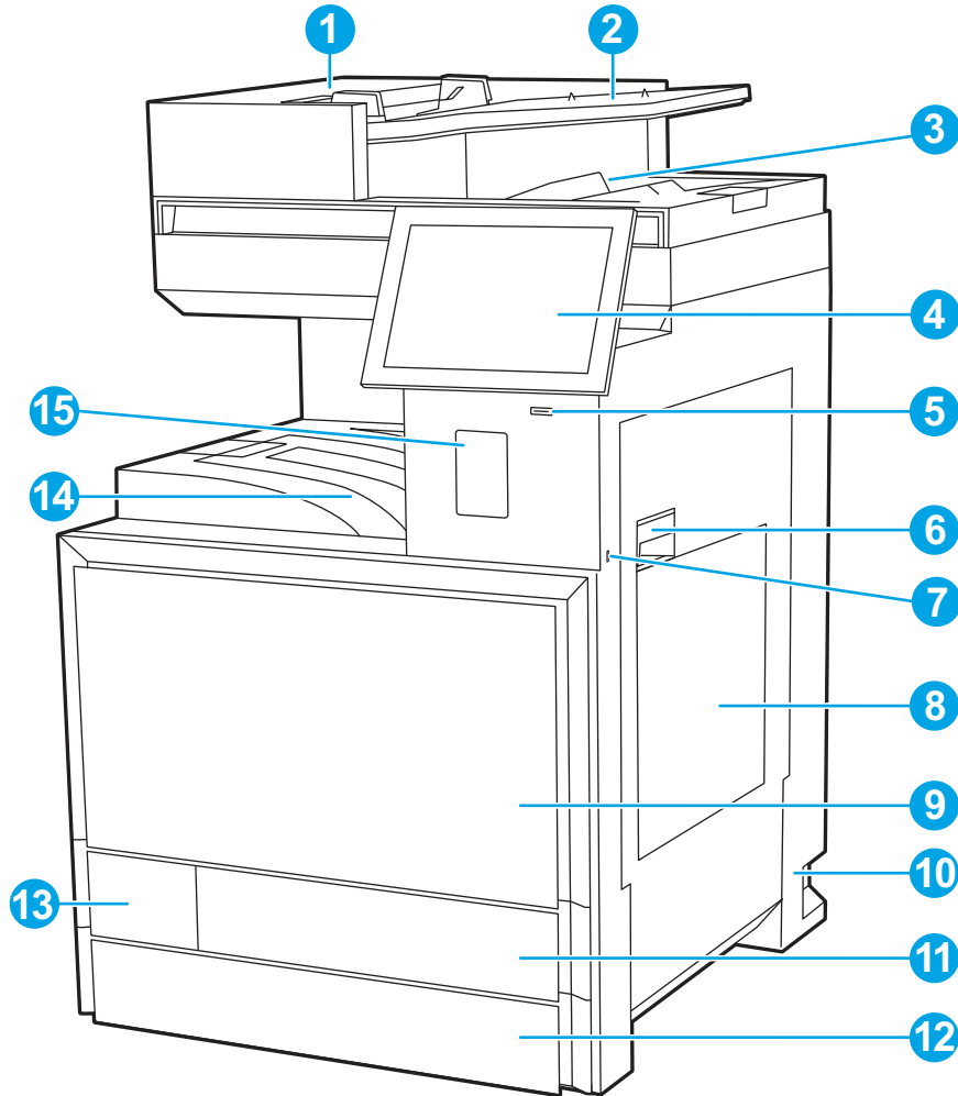
그림 1-6 프린터 전면 보기
