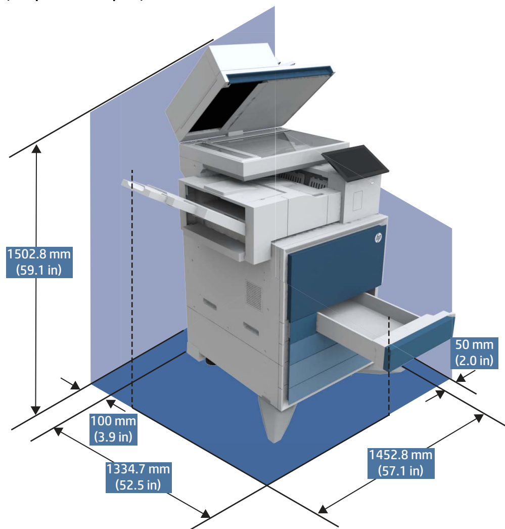
Figura 1-11 Dimensioni della stampante, dell'alimentatore a doppio cassetto e dell'unità di finitura interna (completamente aperti)
