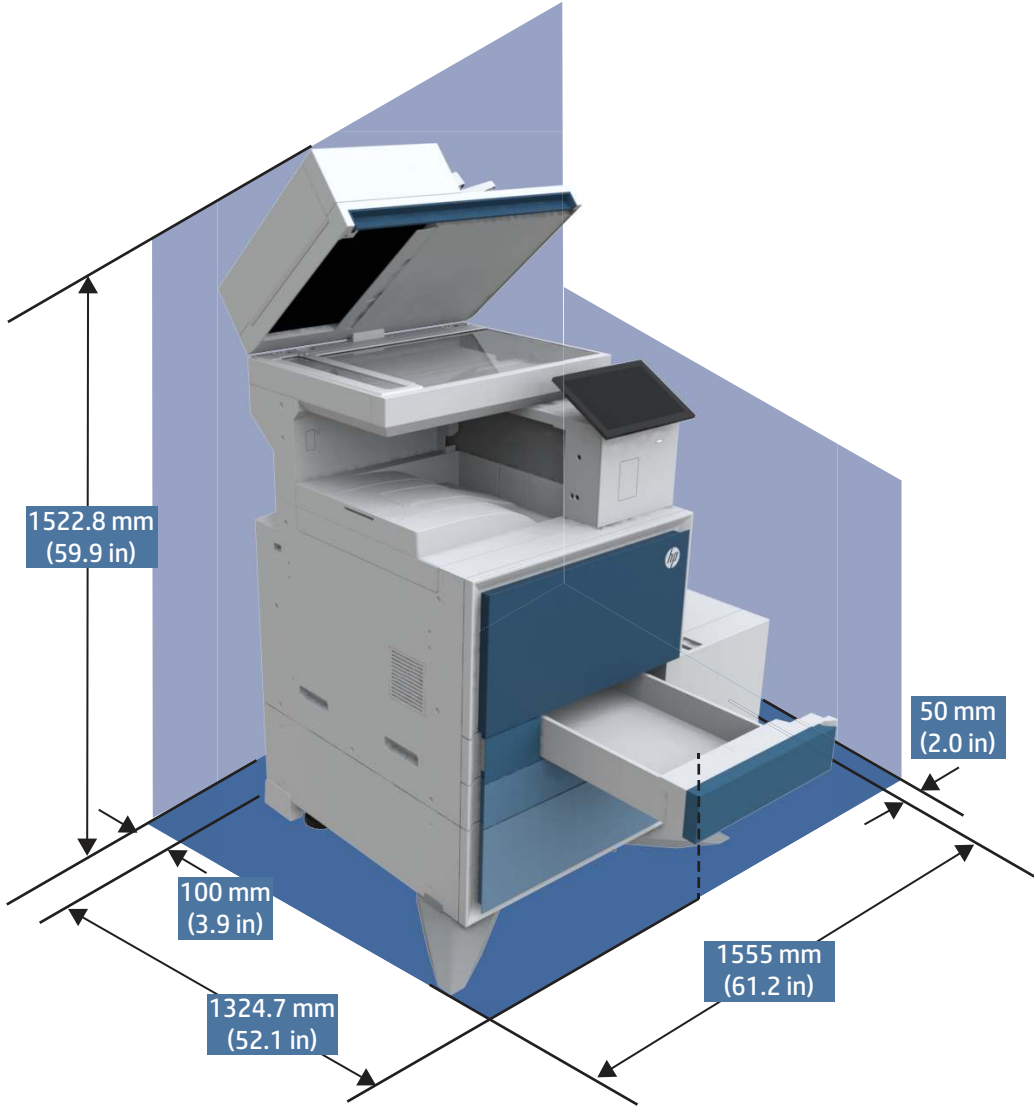
Figura 1-14 Stampante, ingresso ad alta capacità 2K e dimensioni laterali dell'input ad alta capacità (completamente aperte)
