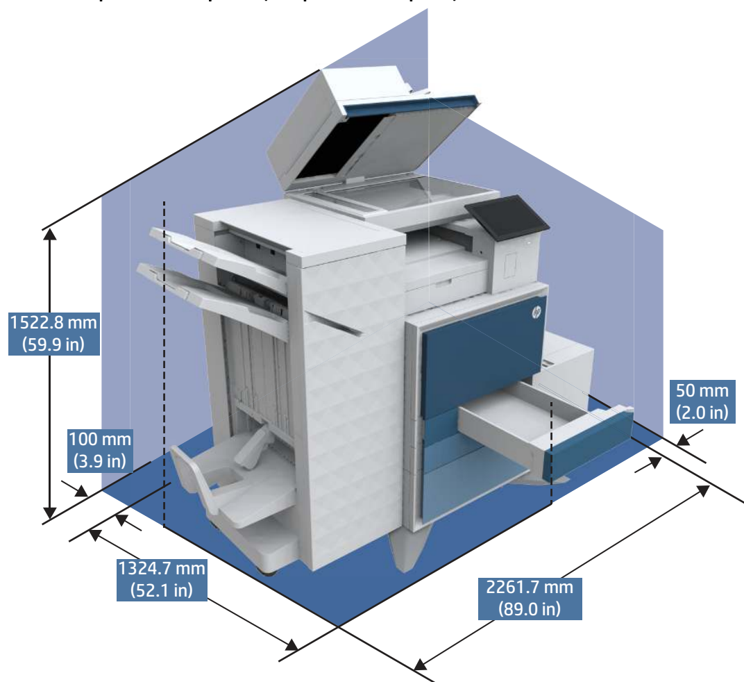
Figura 1-13 Stampante, unità di finitura per opuscoli, alimentazione ad alta capacità 2K e dimensioni laterali di input ad alta capacità (completamente aperte)
