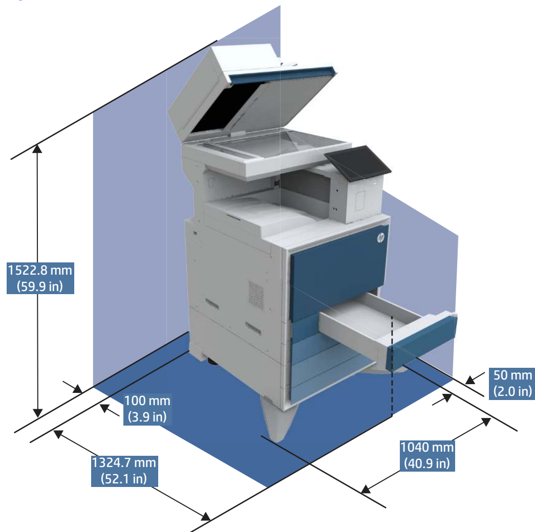
Figura 1-10 Dimensioni della stampante e dell'alimentatore a doppio cassetto (completamente aperti)
