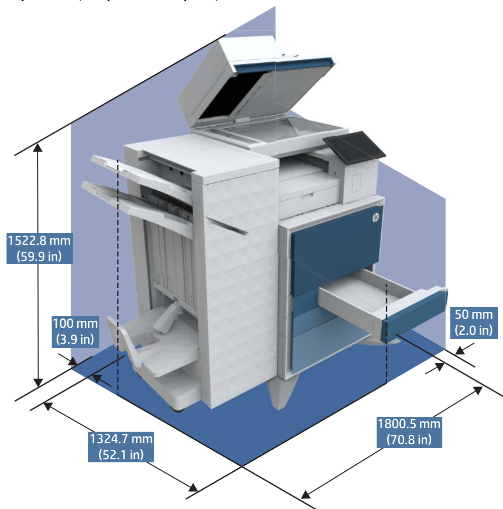
Figura 1-12 Dimensioni della stampante, dell'unità di finitura per opuscoli e dell'alimentatore ad alta capacità 2K (completamente aperte)
