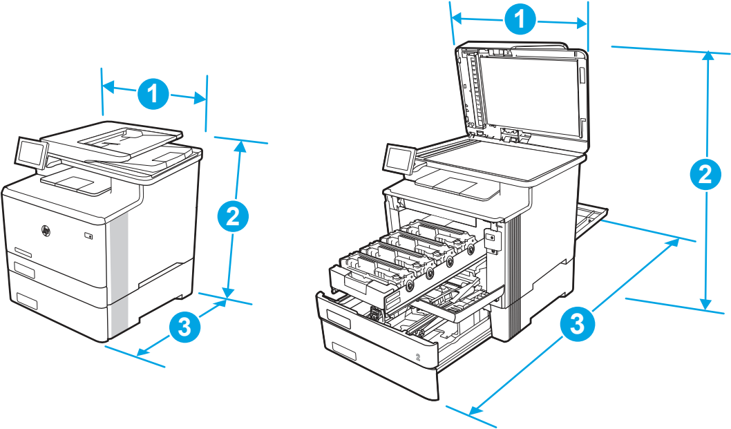
图 1-10 带可选 550 页纸盘的打印机尺寸
