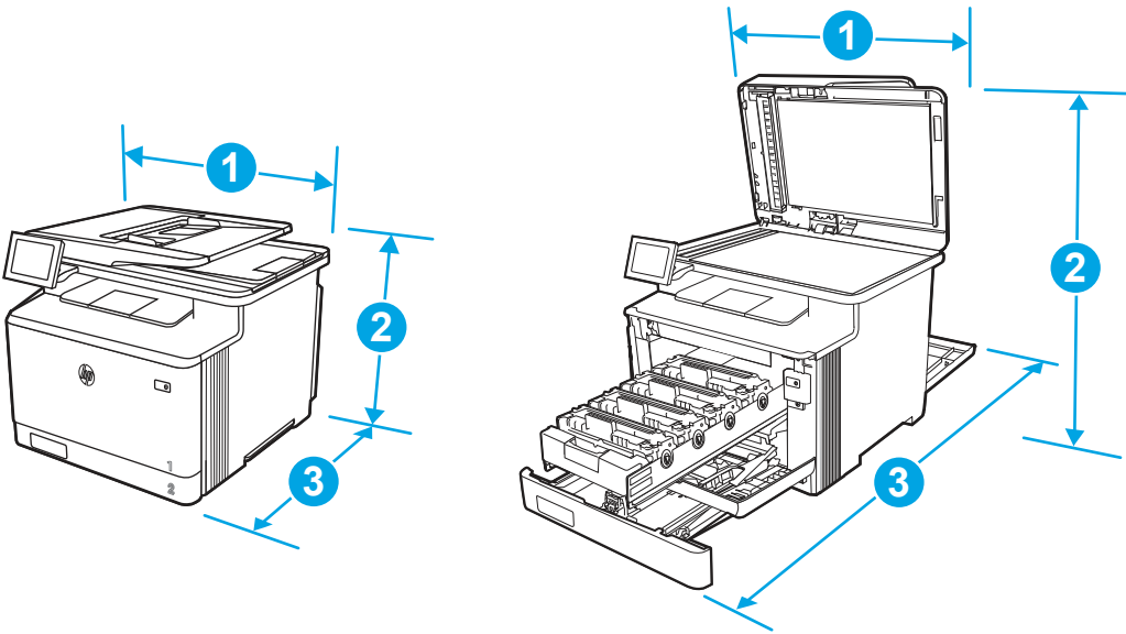
图 1-9 E47528f 型号的尺寸
